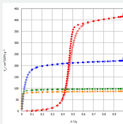
Rôzne merania adsorpcie pár vlákien aktívneho uhlia – H 2 O pri 20 °C (červená), CH 3 OH pri 15 °C (modrá), C 6 H 6 pri 20 °C (zelená) a CCl 4 pri 20 °C (oranžová)
