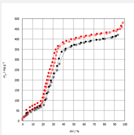
Merania sorpcie vody kovovo-organickým rámcom UiO-66 pri 25 °C (červená) a 40 °C (čierna)
