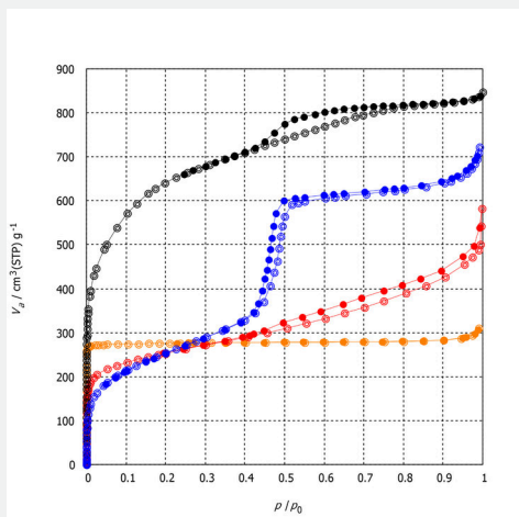
Merania adsorpcie dusíka pri 77 K z aktívneho uhlíkového vlákna (čierna), MCM-41 (modrá), kovovo-organického rámca MIL-160 (oranžová) a katalyzátora PdC (červená)
