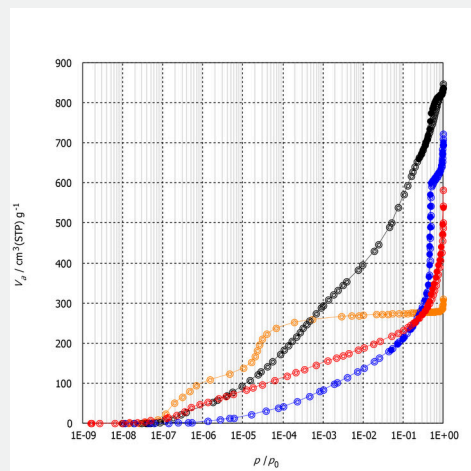
Merania adsorpcie dusíka v logaritmickej mierke pri 77 K z aktívneho uhlíkového vlákna (čierna), zeolitu MCM-41 (modrá), kovovo-organického rámca MIL-160 (oranžová) a katalyzátora PdC (červená)
